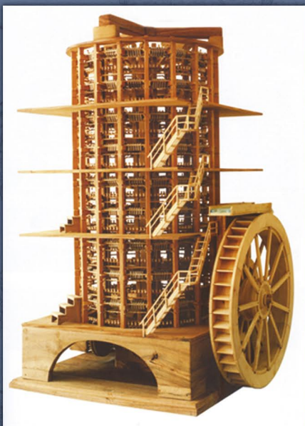
Maquette du moulin à soie de Paolo Micheli (1818). Musée de la Soie Monti, Abbazia Lariana (Italie)
